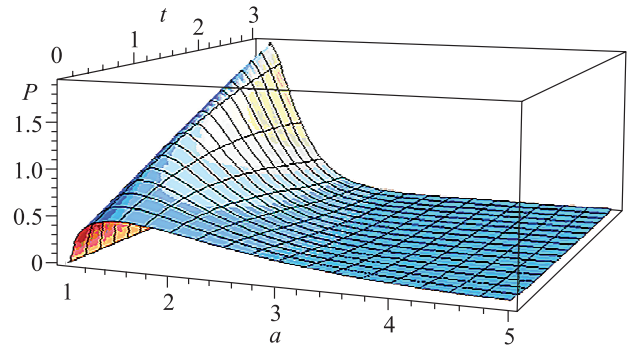
Рис. 2. Динамика распределения мальтузианского параметра при начальном \Gamma -распределении.
